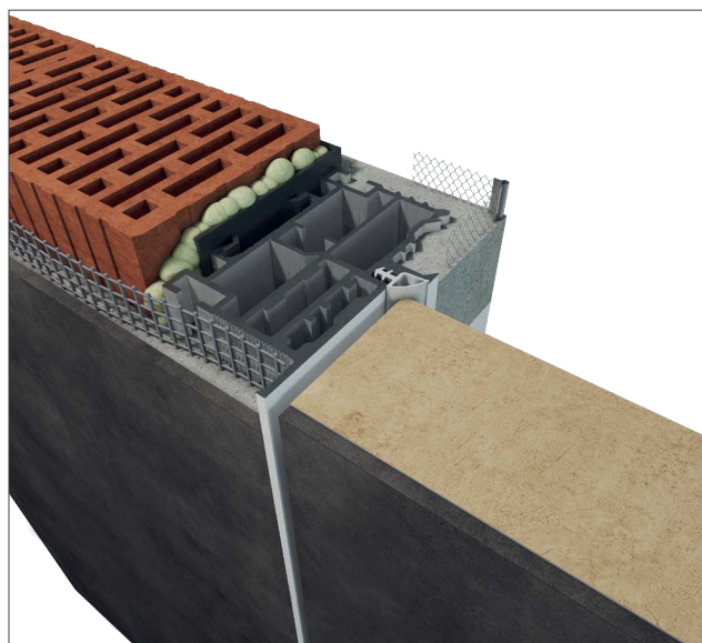
DVEŘE SOP CZ VNEJŠÍ
