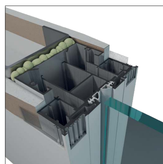
4. HLINÍKOVÁ ZARÁŽKA (B01-B06)
