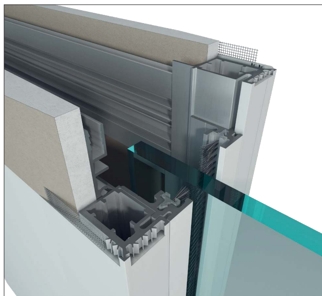
BEZZÁRUBŇOVÁ KAZETA B 01CZ PRO SKLENĚNÁ KŘÍDLA
