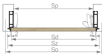
SKRYTÁ ZÁRUBEŇ PRO VESTAVĚNÉ SM CZ
