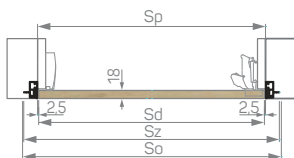
ZÁRUBEŇ PRO VESTAVĚNÉ SMP CZ
