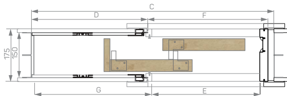
TELESKOPICKÁ ZÁRUBŇOVÁ KAZETA FT CZ PRO DŘEVĚNÁ KŘÍDLA
