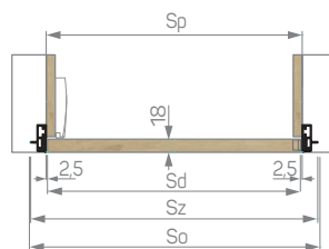
SKRYTÁ ZÁRUBEŇ PRO VESTAVĚNÉ SMP CZ
