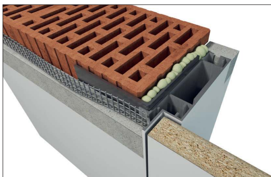
SKRYTÁ ZÁRUBEŇ PRO VESTAVĚNÉ SM CZ
