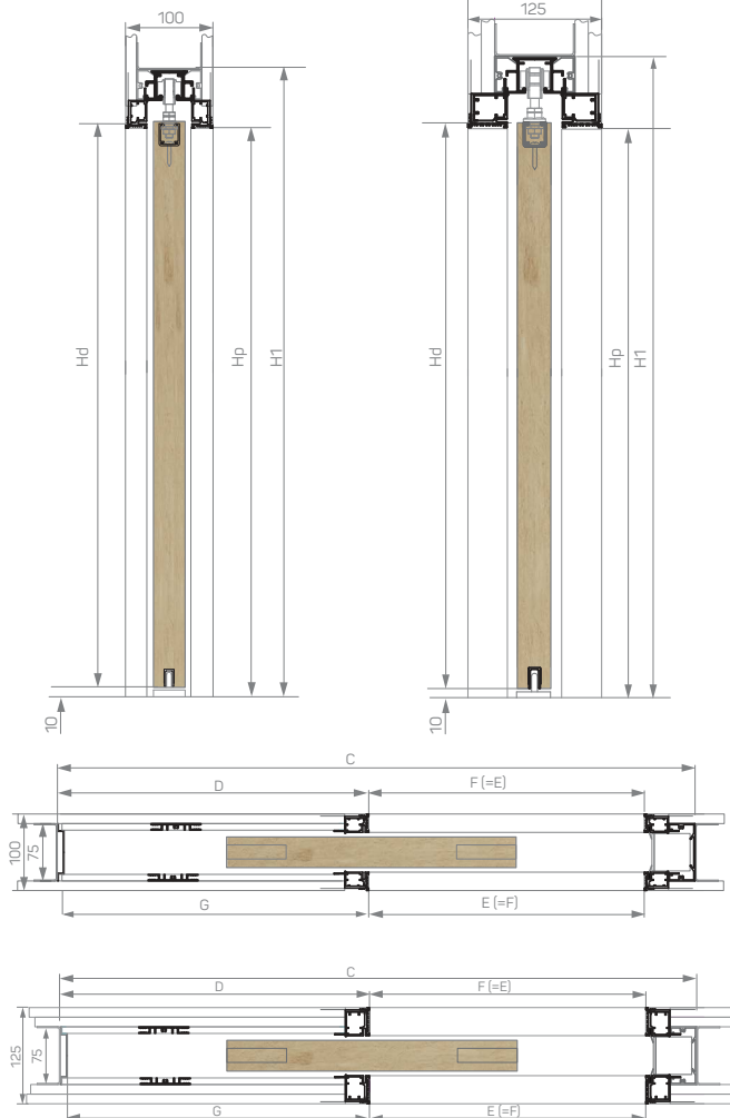
B 01D (100 MM)
