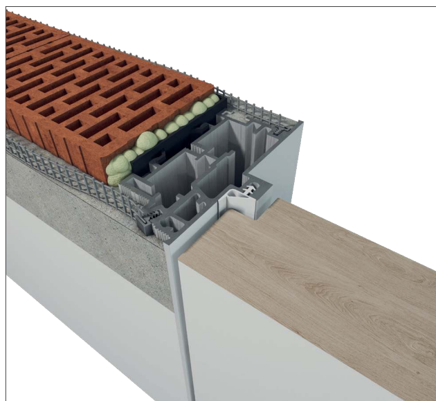
DVEŘE SPN CZ D VNĚJŠÍ
