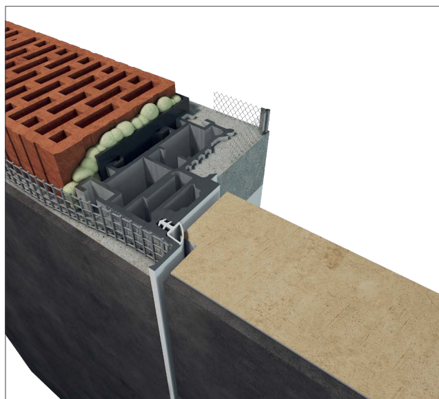
DVEŘE SOP CZ VNITŘNÍ
