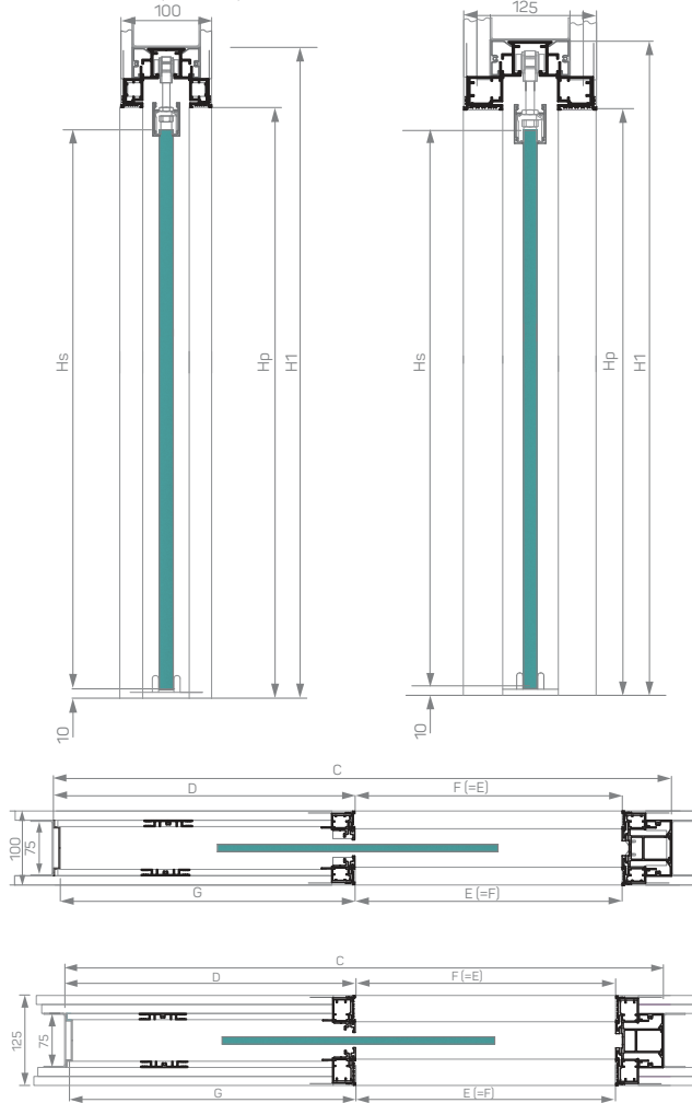
B 01V (100 MM)
