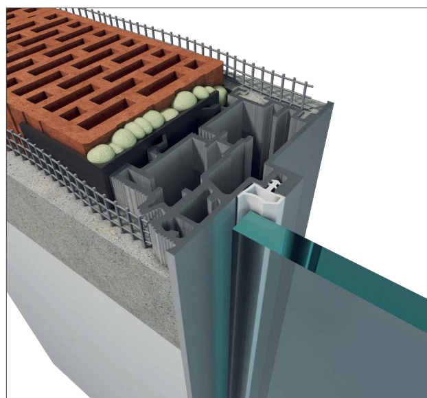
DVEŘE SPN CZ V VNĚJŠÍ
