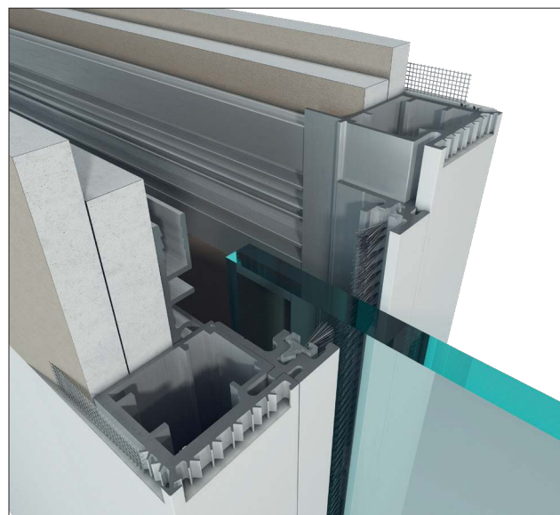
BEZZÁRUBŇOVÁ KAZETA STROPNÍ B 05 CZ PRO SKLENĚNÁ KŘÍDLA
