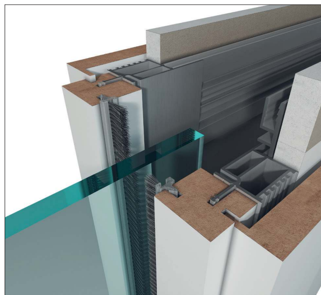
ZÁRUBŇOVÁ KAZETA F CZ PRO SKLENĚNÁ KŘÍDLA
