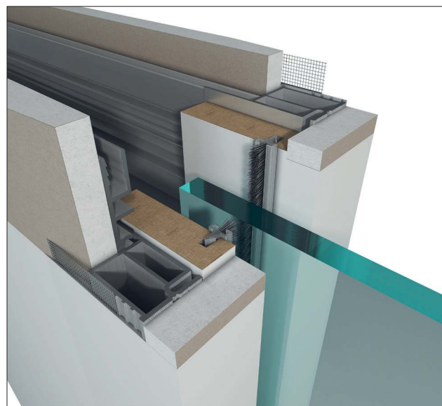
BEZZÁRUBŇOVÁ KAZETA B 01eco CZ PRO SKLENĚNÁ KŘÍDLA
