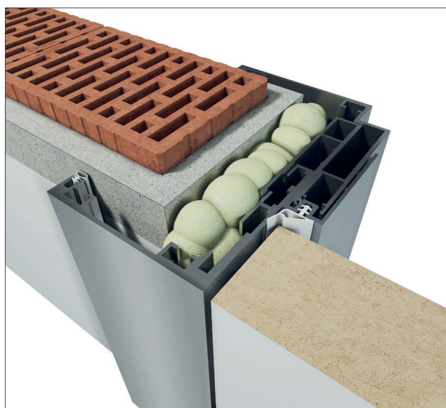
DVEŘE LP CZ D DŘEVĚNÉ KŘÍDLO
