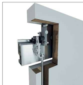
4. ZÁMEK STV NAHOŘE
